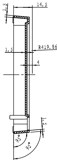
剖面 B-B
