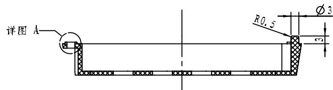
剖面 A-A
