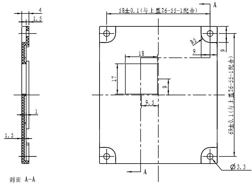
剖面 A-A
