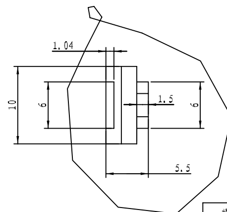
细节 A 比例 3:1
