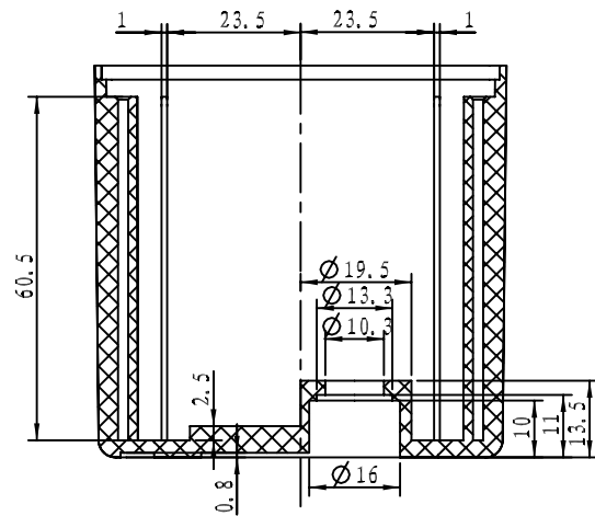
截面 B-B
