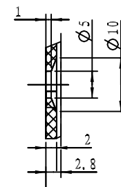
剖面 A-A
