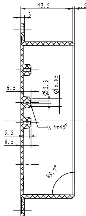
截面 B-B
