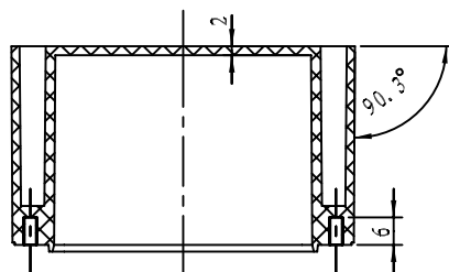
截面 A-A
