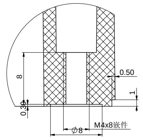
局部视图 C 比例 4:1
