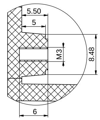
局部视图 E 比例 3:1
