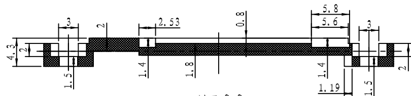
剖面 C-C
