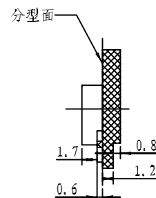
剖面 D-D
