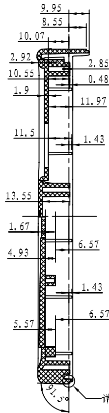
剖面 A-A
