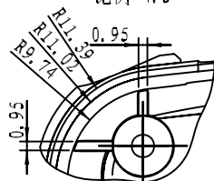
细节 B 比例 2:1
