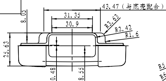
背面(此面做顶杆)
