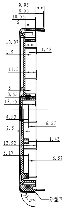
剖面 A-A
