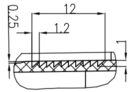
视图C 比例 2:1
