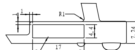
此做镶块 细节 A 比例 2:1
