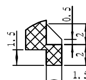
细节 D 刻度 4:1
