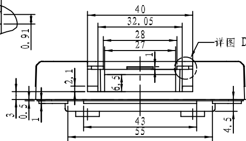
细节 D 比例 4:1
