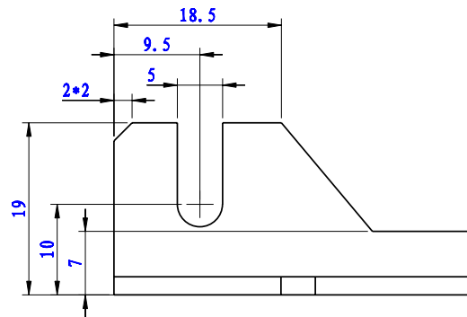
细节 B 比例 2:1
