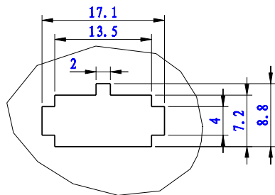
细节 A 比例 2:1
