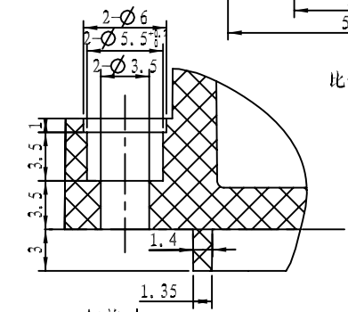
细节 A 比例 3:1
