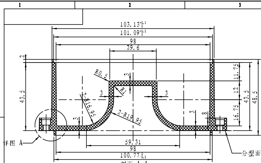
剖面 A-A 正面 (此面做顶杆)
