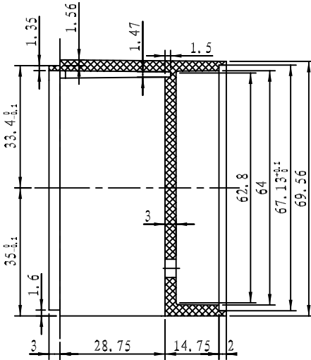
剖面 B-B
