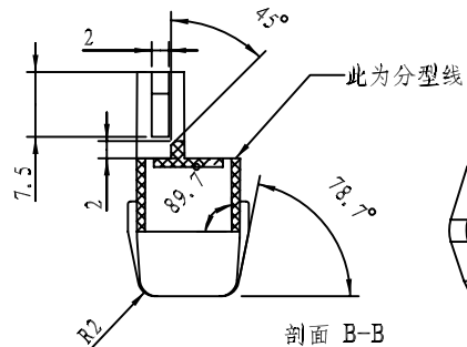
剖面 B-B
