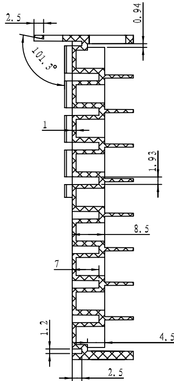
剖面 C-C
