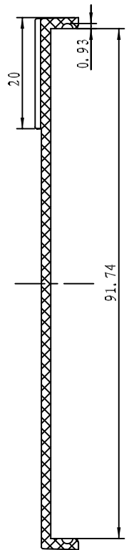
剖面 B-B
