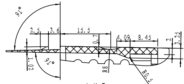
细节 D 刻度 2:1
