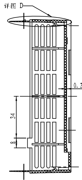
截面 A-A
