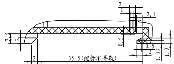
细节 E 刻度 2:1
