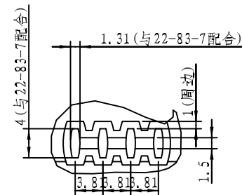
细节 C 刻度 2:1
