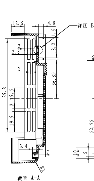
截面 A-A
