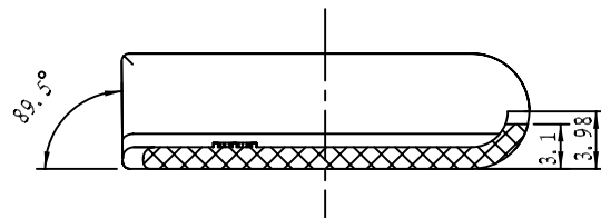
截面 B-B
