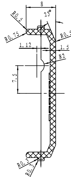
截面 A-A
