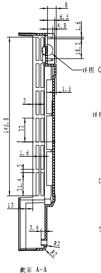
截面 A-A
