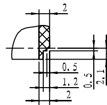
细节 A 比例 2:1
