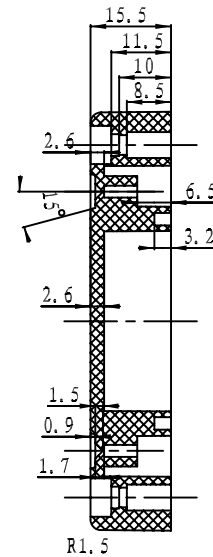
剖面 A-A
