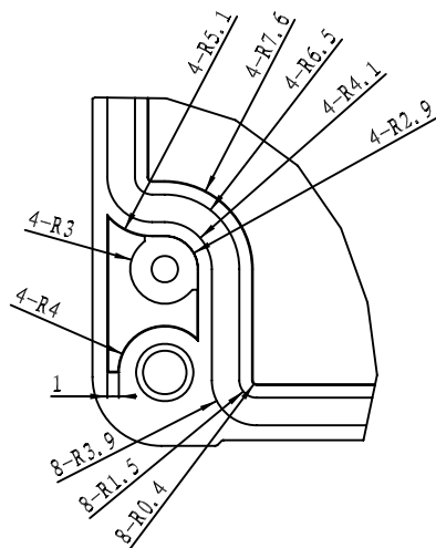
细节 B 比例 2:1
