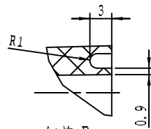
细节 B 比例 2:1
