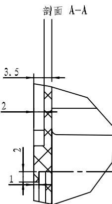
细节 A 比例 2:1
