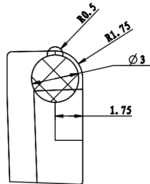
剖面 A-A
