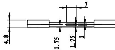
剖面 C-C
