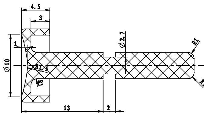
截面 A-A
