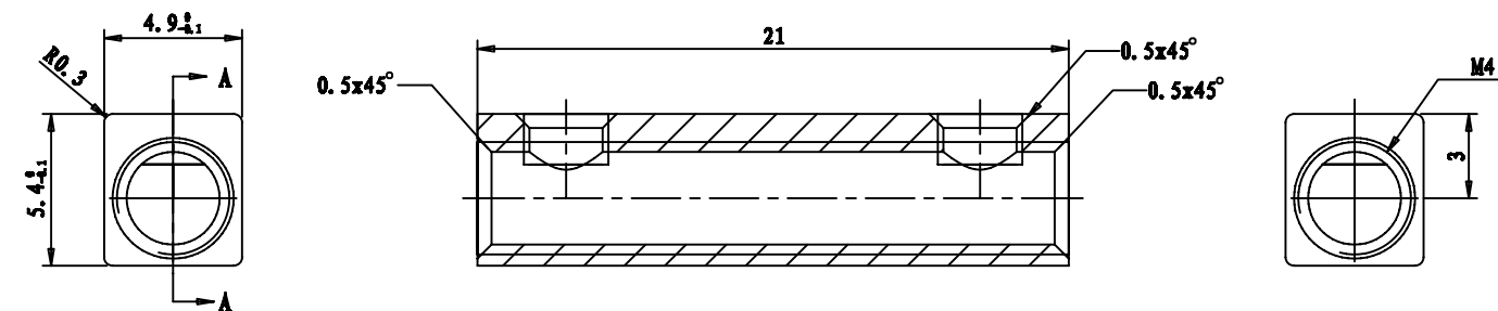
截面 A-A
