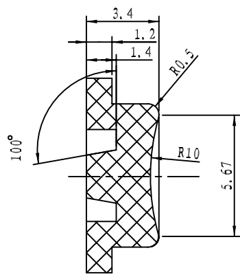
剖面 D-D
