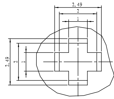
剖面 D-D
