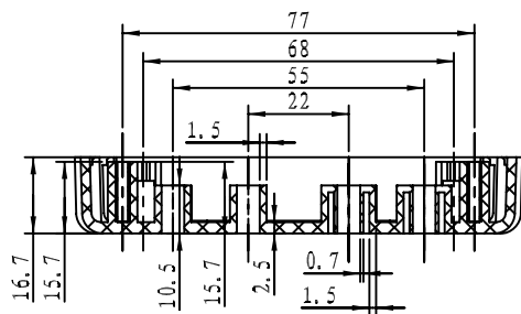
剖面 H-H
