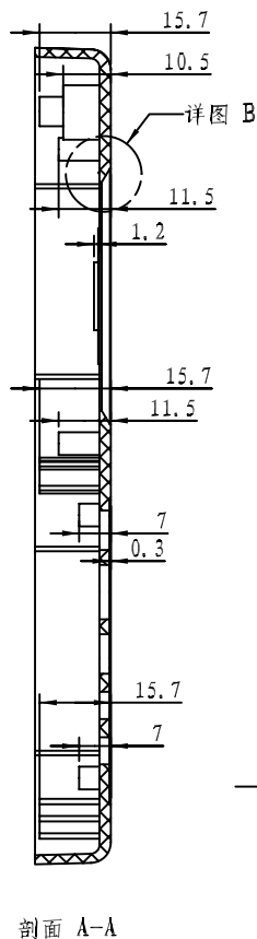
剖面 A-A
