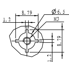
细节 A 比例 2:1
