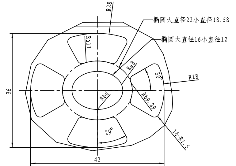
细节 A 比例 2:1
