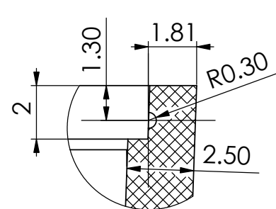
局部视图 E 比例 5:1
