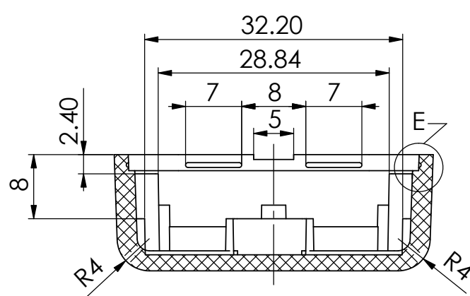
剖面 B-B
