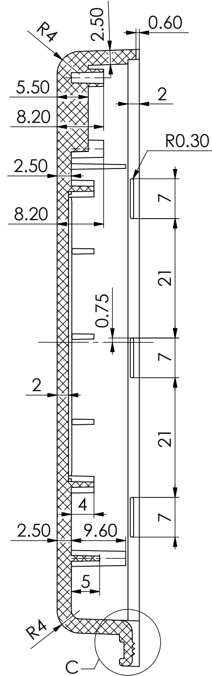
剖面 A-A
