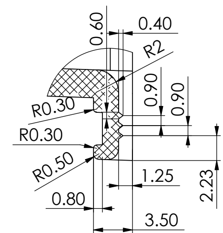
局部视图 C 比例 3:1
