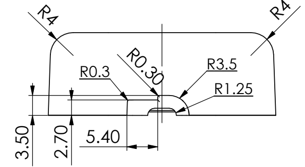
A向视图
