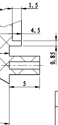
细节 A 比例 4:1
