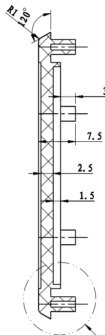
剖面 A-A
