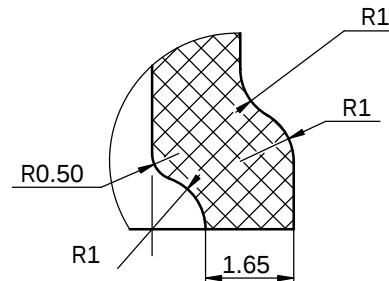
局部视图 B 比例 10:1
