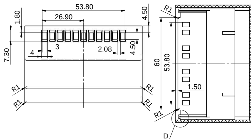
剖面 B-B
