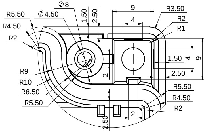
局部视图 C 比例 3:1
