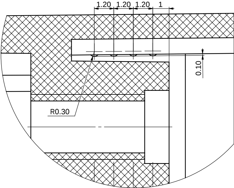
局部视图 F 比例 10:1
