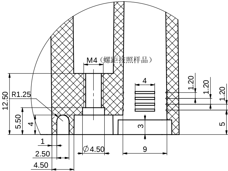
局部视图 D 比例 3:1
