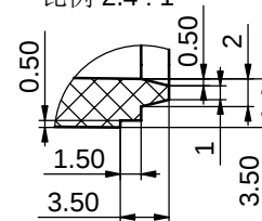
局部视图 C 比例 2.4 : 1
