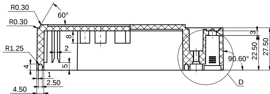
剖面 B-B
