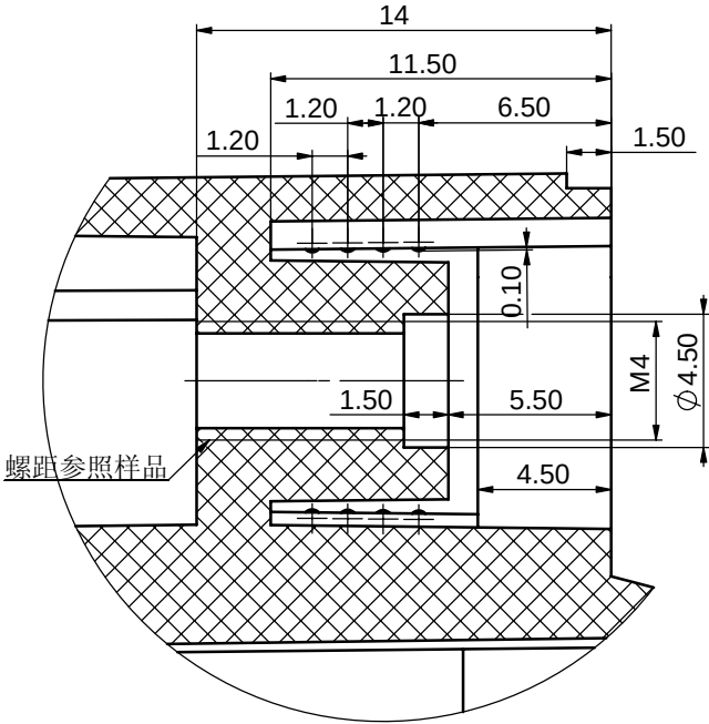
局部视图 E 比例 5:1
