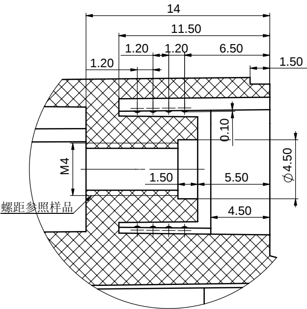
局部视图 E 比例 5:1
