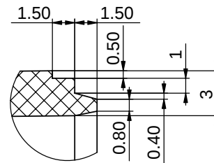
局部视图 D 比例 4 : 1
