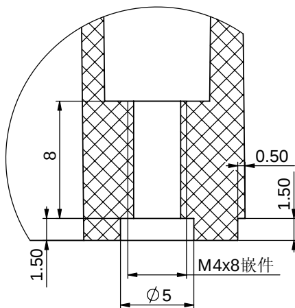
局部视图 C 比例 4 : 1
