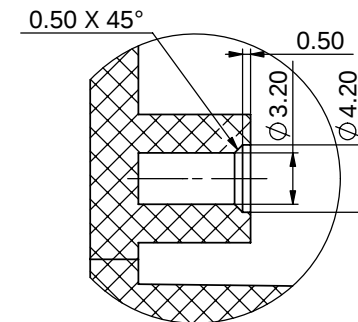
局部视图 E 比例 3 : 1
