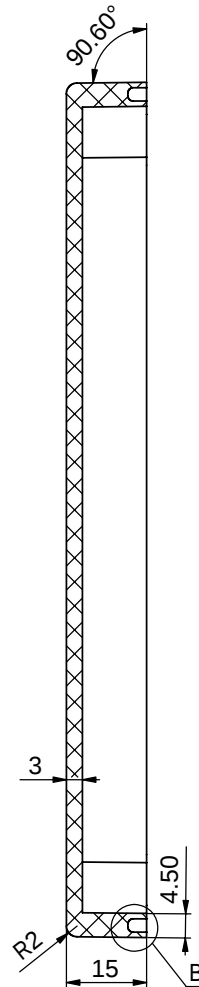
剖面 A-A
