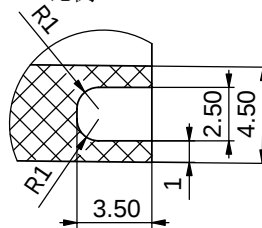
局部视图 B 比例 4:1
