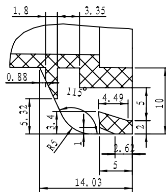
细节 D 比例 5:2
