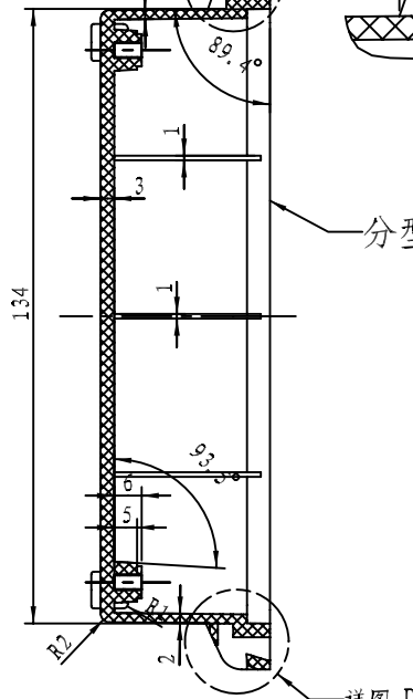
截面 A-A
