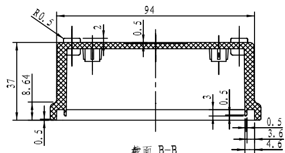
截面 B-B
